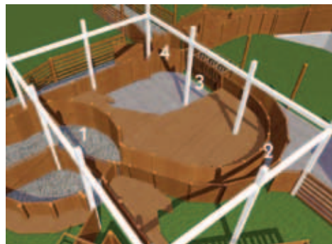
VISTA DA ÁREA DE MANEJO INTENSIVO NUM CURRAL, ONDE: 1= SERINGA COM PORTEIRAS GIRATÓRIAS, 2= BRETE (CORREDOR ESTREITO QUE LIGA A SERINGA AO TRONCO DE CONTENÇÃO E BALANÇA, TAMBÉM CONHECIDO COMO TRONCO COLETIVO) EM CURVA, 3= TRONCO DE CONTENÇÃO INDIVIDUAL; 4= APARTADOR TIPO "OVO"
